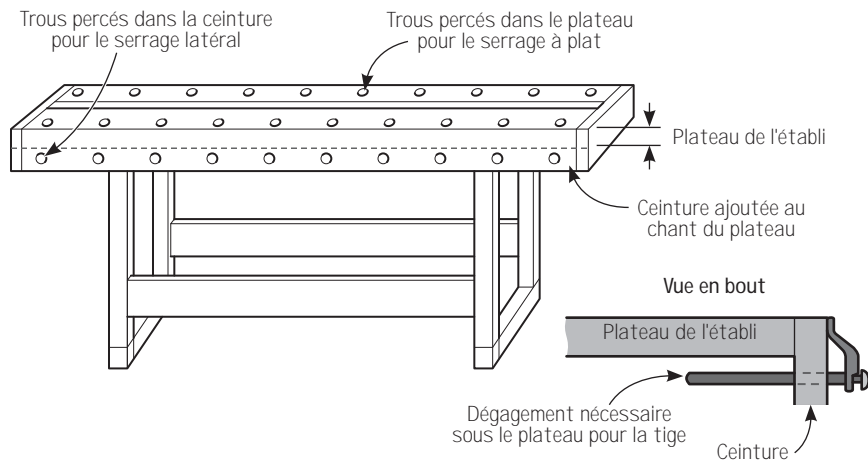
Figure 1 : Exigences concernant l'établi.
