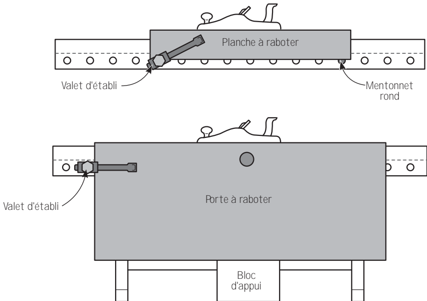
Figure 2 : Utilisations typiques du valet d'établi pour le serrage latéral
