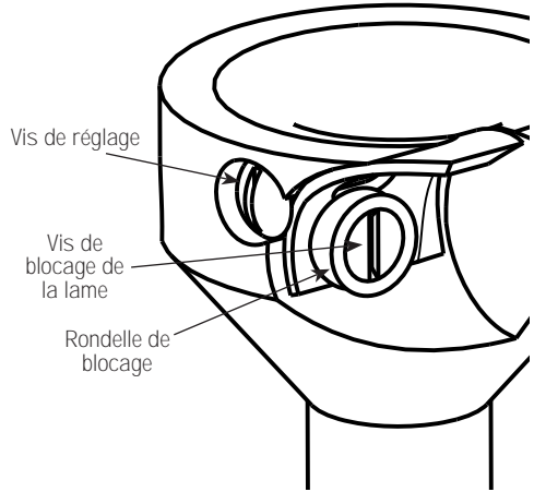
Figure 1 : Réglage de la lame
