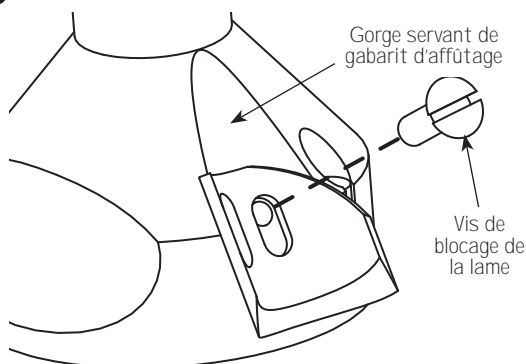
Figure 5 : Montage de la lame pour l'affûtage
