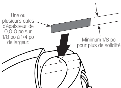
Figure 3 : Calage de la lame pour réduire l'épaisseur du copeau
