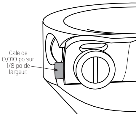
Figure 2 : Calage de la lame pour augmenter le diamètre du tenon
