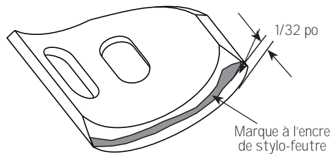
Figure 7 : Détail de la lame
