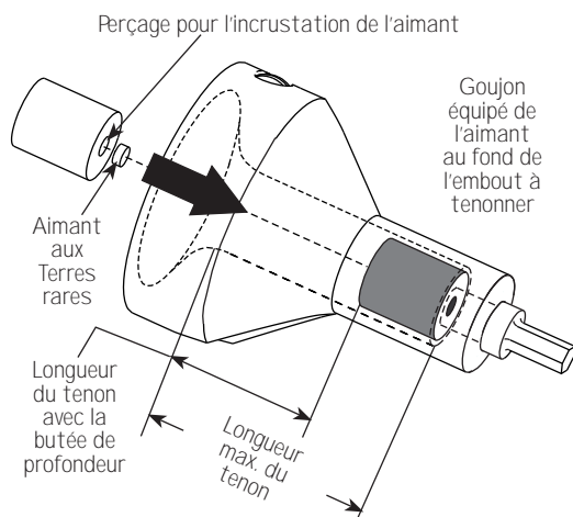
Figure 4 : Butée de profondeur
