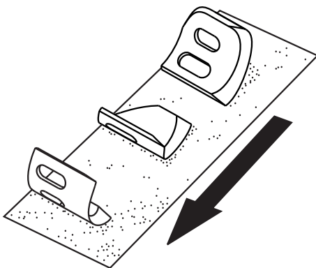
Figure 8 : Élimination du morfil
