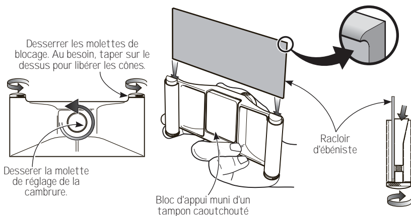
Figure 1 : Installation du racloir dans le porte-racloir
