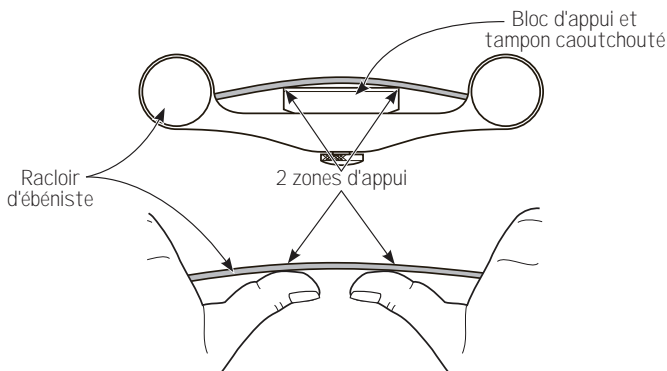
Figure 3 : Le bloc d'appui soutient le racloir comme le feraient les pouces.
