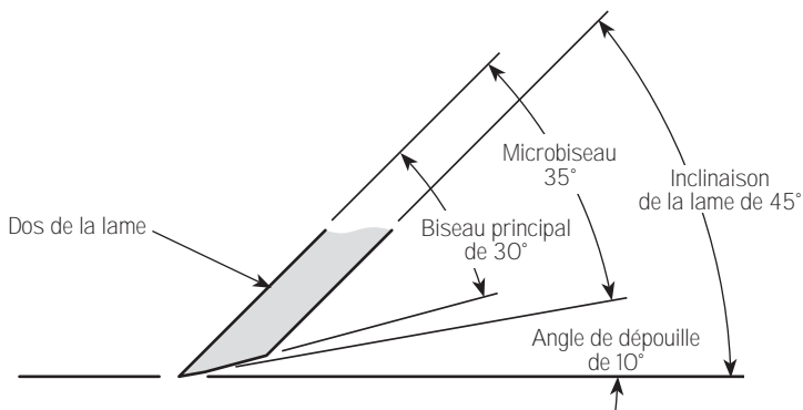
Figure 4 : Lame avec un microbiseau
