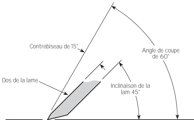
Figure 5 : Lame avec un contrebiseau
