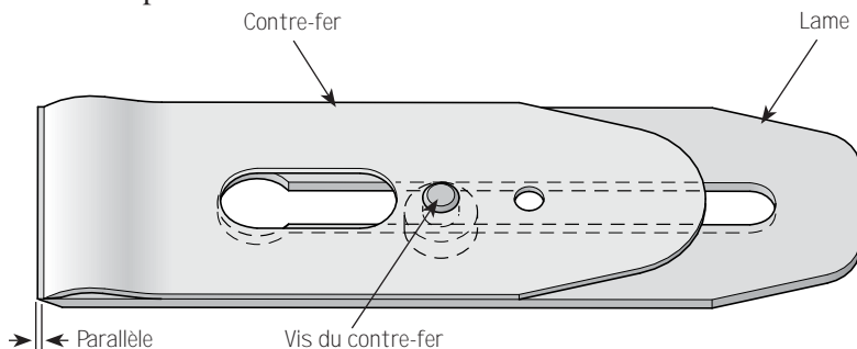
Figure 2 : Ensemble lame et contre-fer
