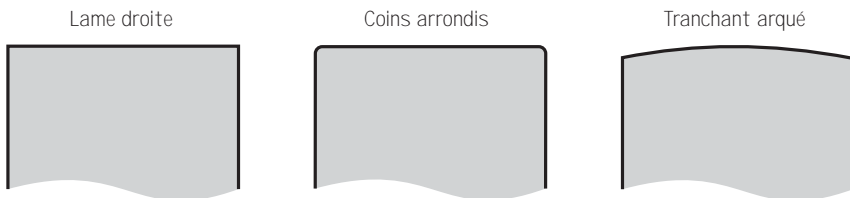
Figure 6 : Formes de lames
